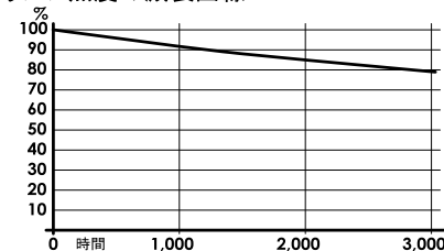
ランプ照度の減衰曲線
